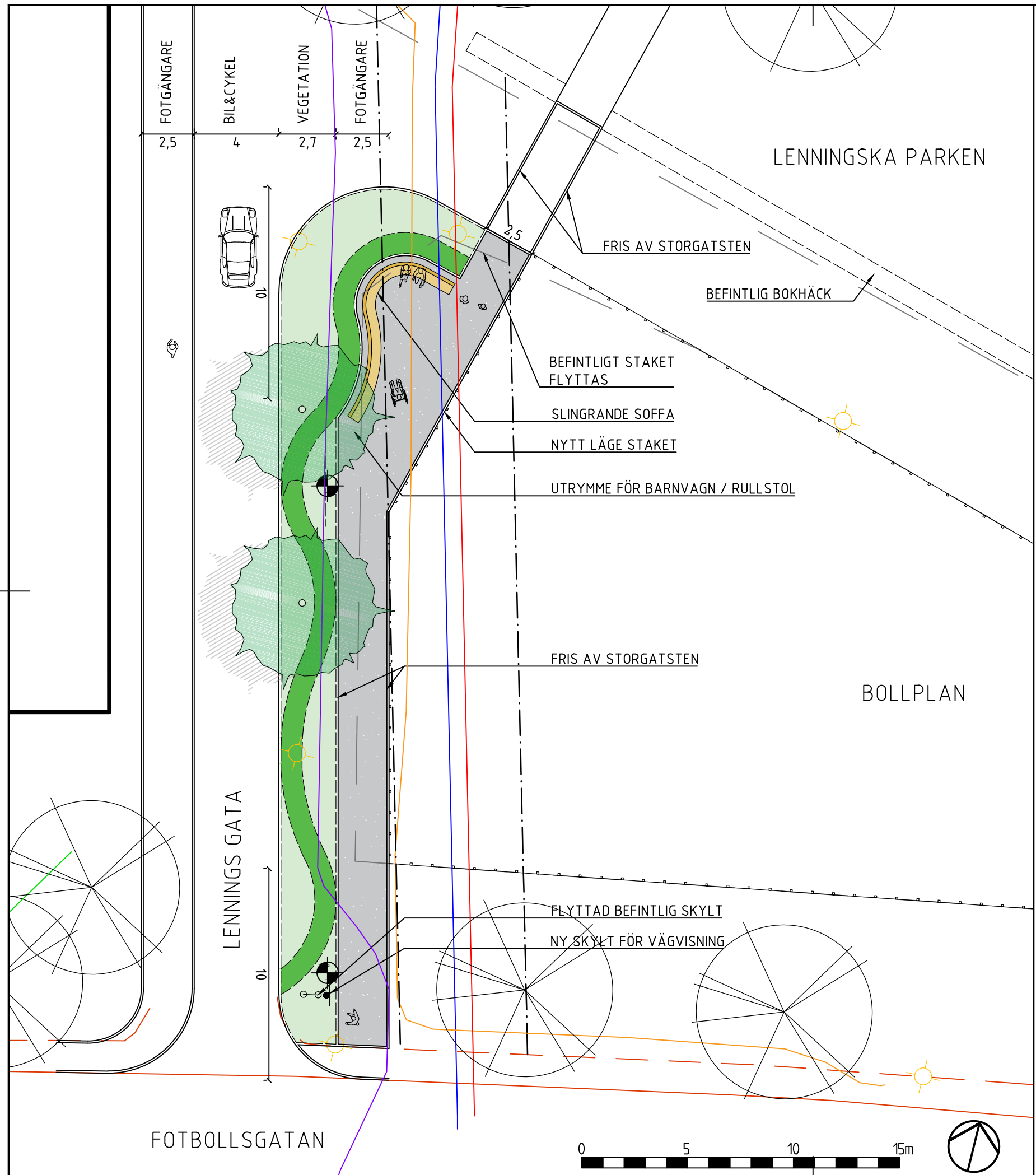
SLINGRANDE SOFFA
